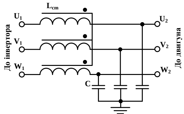
Рисунок 3 – Синфазний фільтр
