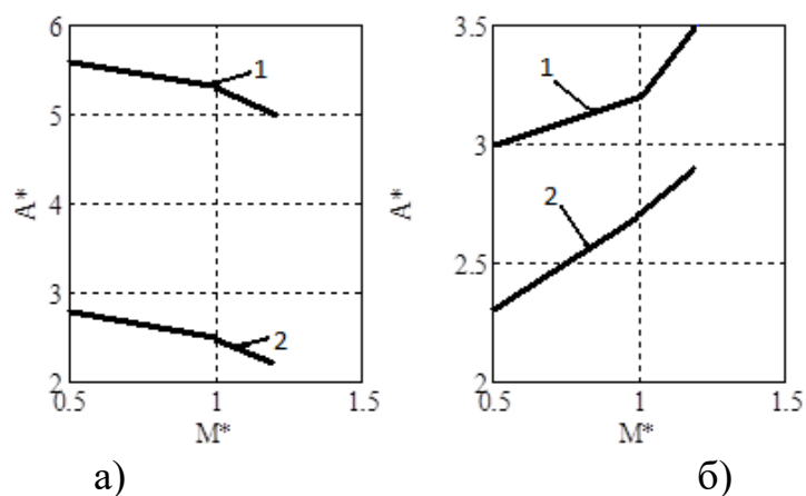
Рисунок 3 – Графіки зміни амплітуди коливань в тяговому органі : 1 – розташування двох електродвигунів в головній частині конвеєра; 2 – розташування по одному електродвигуну в головній та хвостовій частині конвеєрної установки
