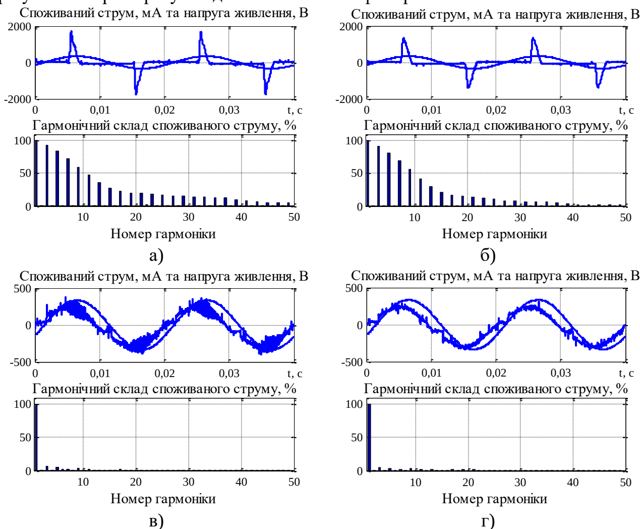
Рис. 2. Графіки напруги живлення, споживаного струму та діаграми його гармонічного складу: а) – без ЕМІ фільтру та без PFC; б) – з ЕМІ фільтром та без PFC; в) – без ЕМІ фільтру та з PFC; г) – з ЕМІ фільтром та з PFC
