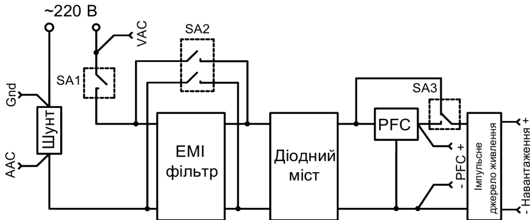
Рис. 1. Спрощена електрична принципова схема лабораторного стенду
